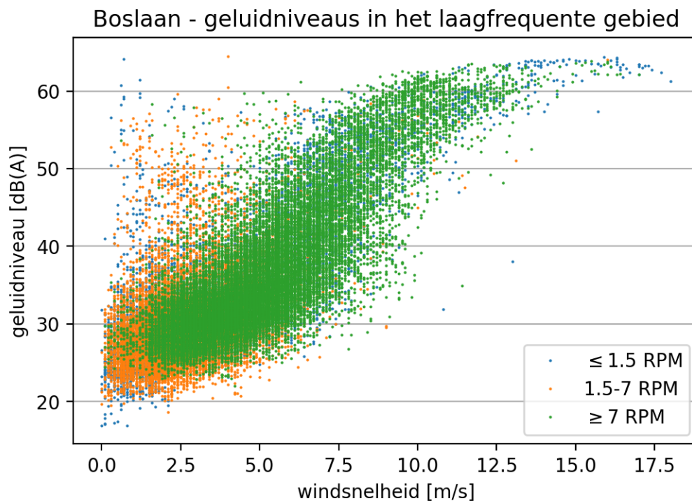
figuur 30: spreidingsdiagram voor de geluidniveaus in het laagfrequente gebied
